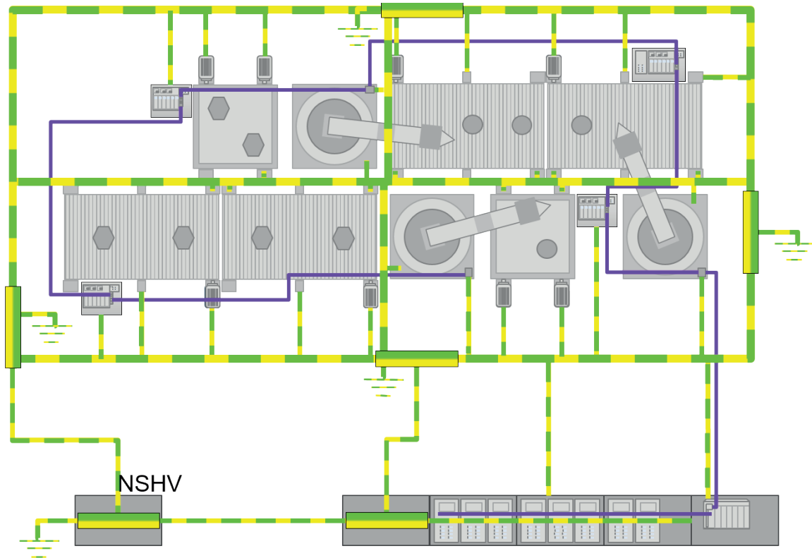
Fig. 15: Equipotential bonding and grounding
